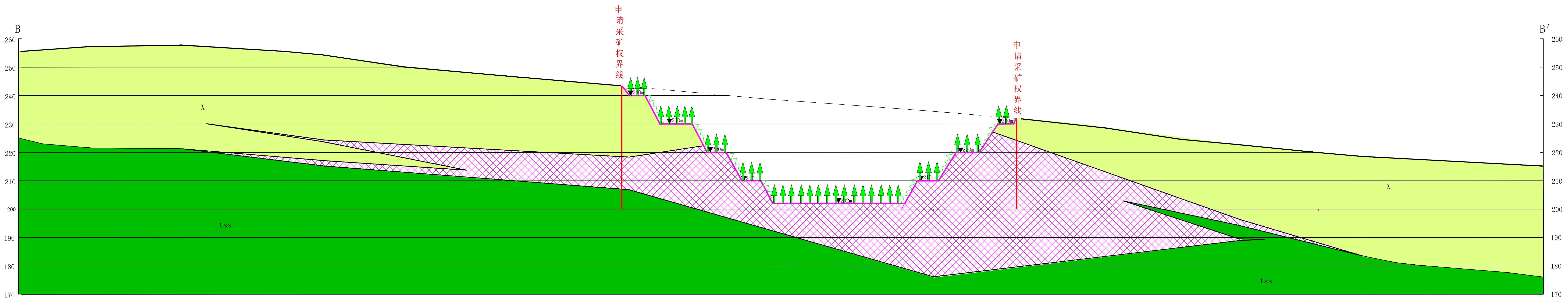
III采区B-B' 开采终了治理复垦剖面图 比例尺 1:1000
